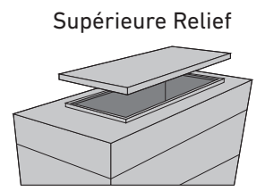
Supérieure Relief Ouverture 76 x 172 cm 1 Dalle 94 x 174 cm
