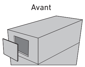
Avant Ouverture 59 x 80 cm Porte 60 x 83 cm
